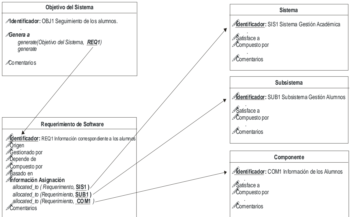
Figura 7.1 Evaluación de Impacto- Cambio de un Objetivo del Sistema
