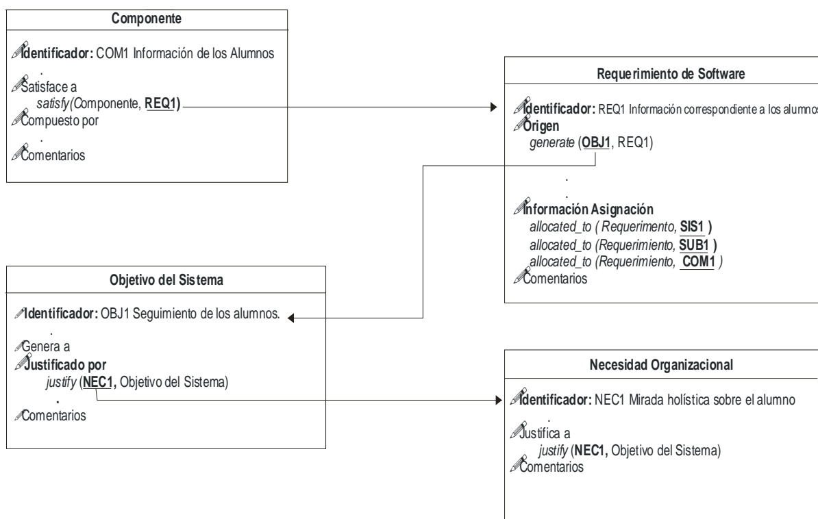
Figura 7.2 Información Asignación Requerimientos
