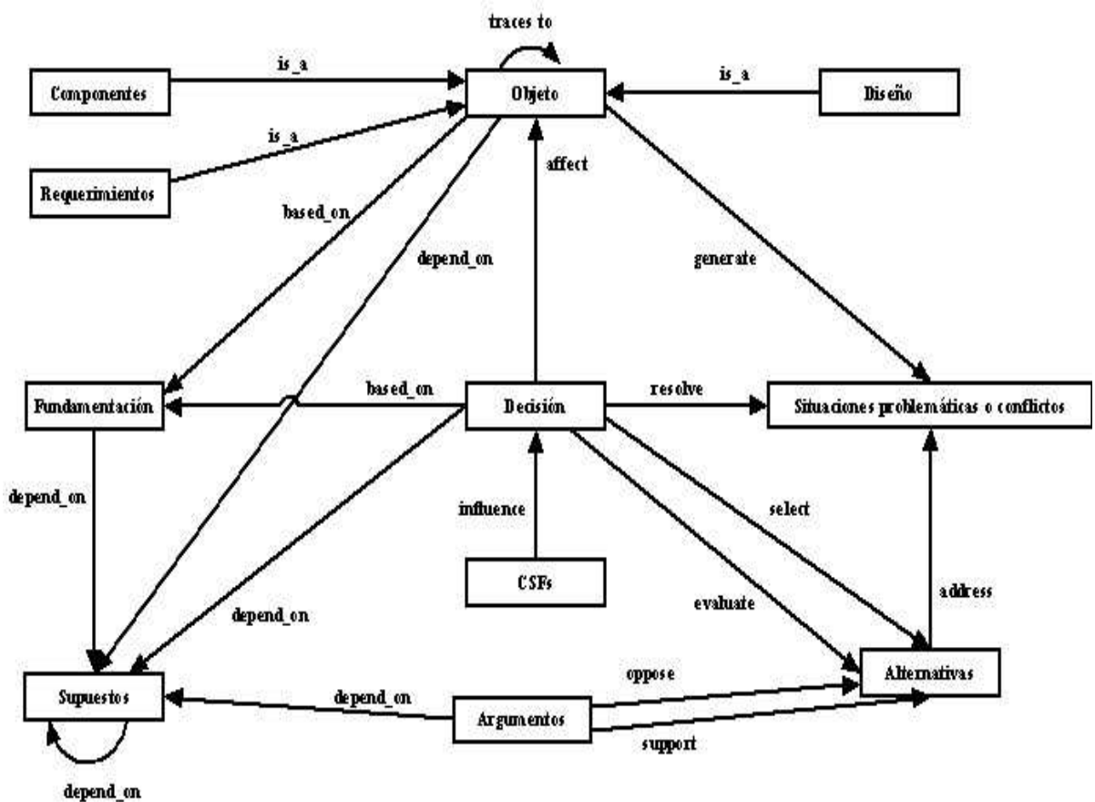
Figura 5.3 Submodelo Fundamentación [Ramesh et. al, 2001].
