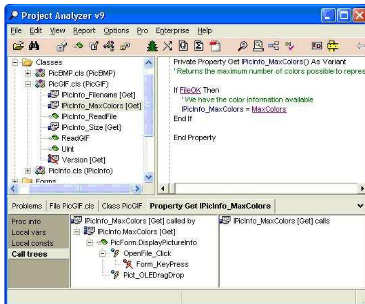
Figura 3.6: Aivosto Project Analyzer
