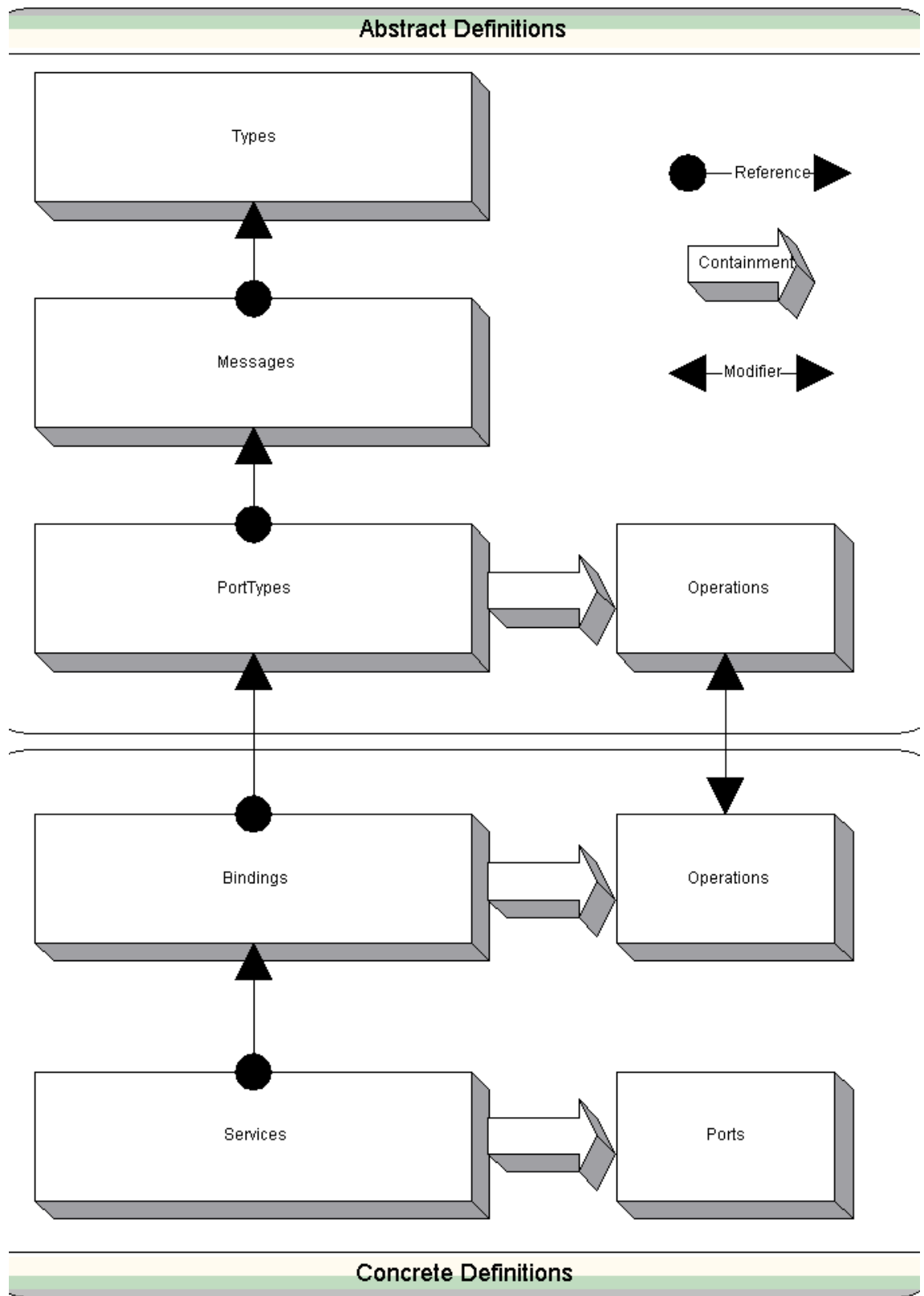
Diagrama de un documento WSDL
