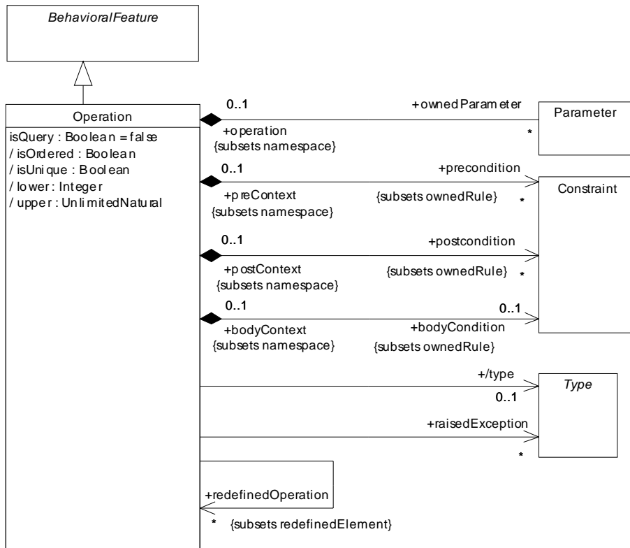
Diagrama de clases de Operations
