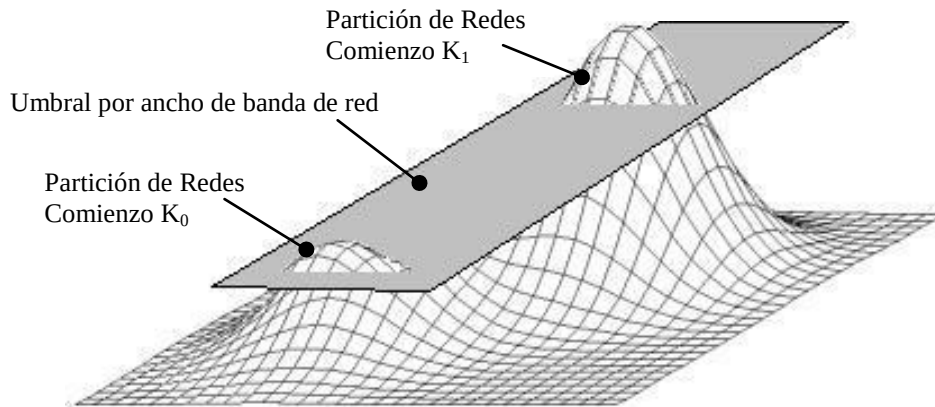
Figura 38. Espacio de todas las posibles soluciones con umbral por enlace de red
