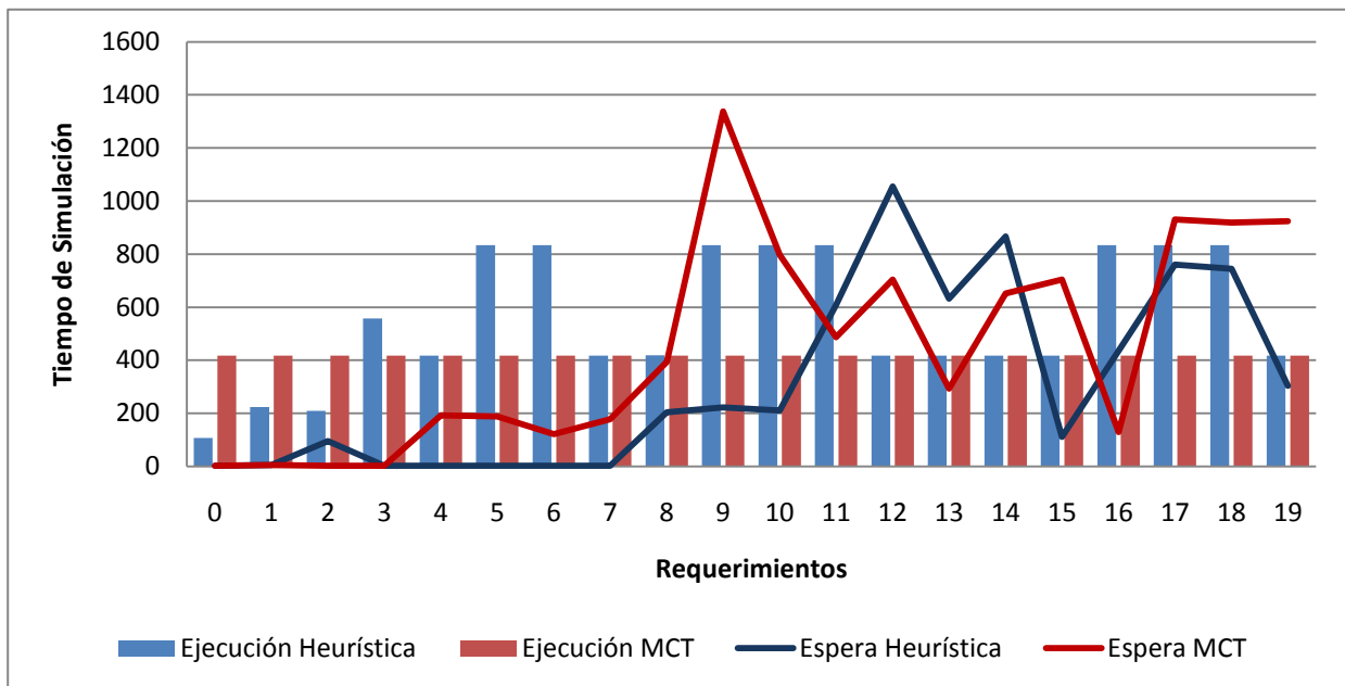
Figura 50. Ejecución Heurística y MCT con respectivos tiempos de espera
