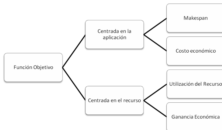
Figura 31. Funciones objetivo
