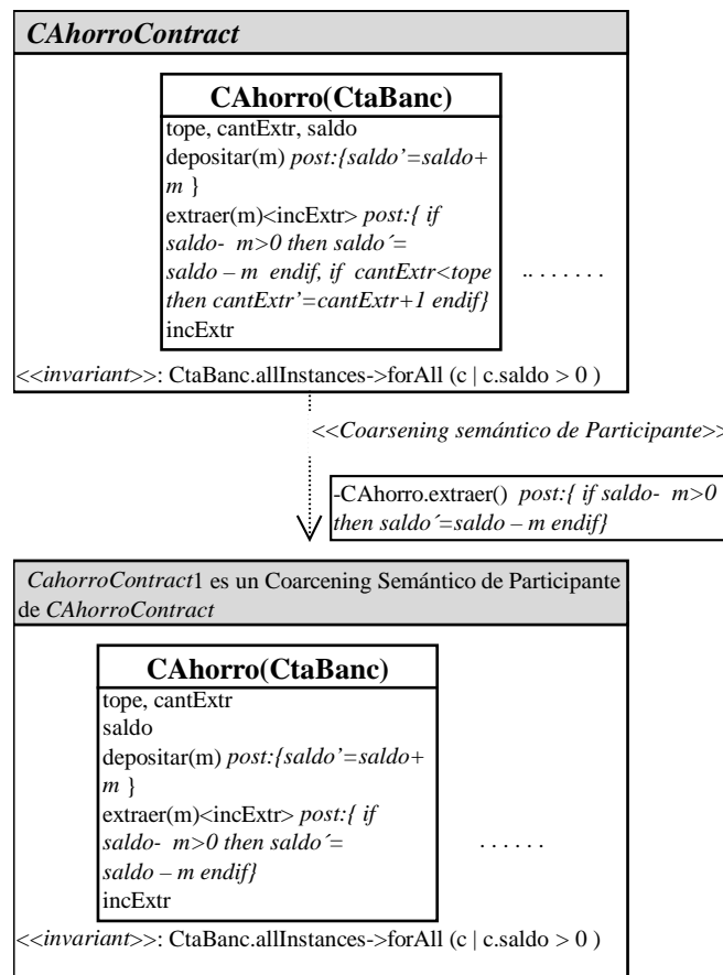
Fig. 4.3. Un ejemplo de Coarsening Semántico de Participante
