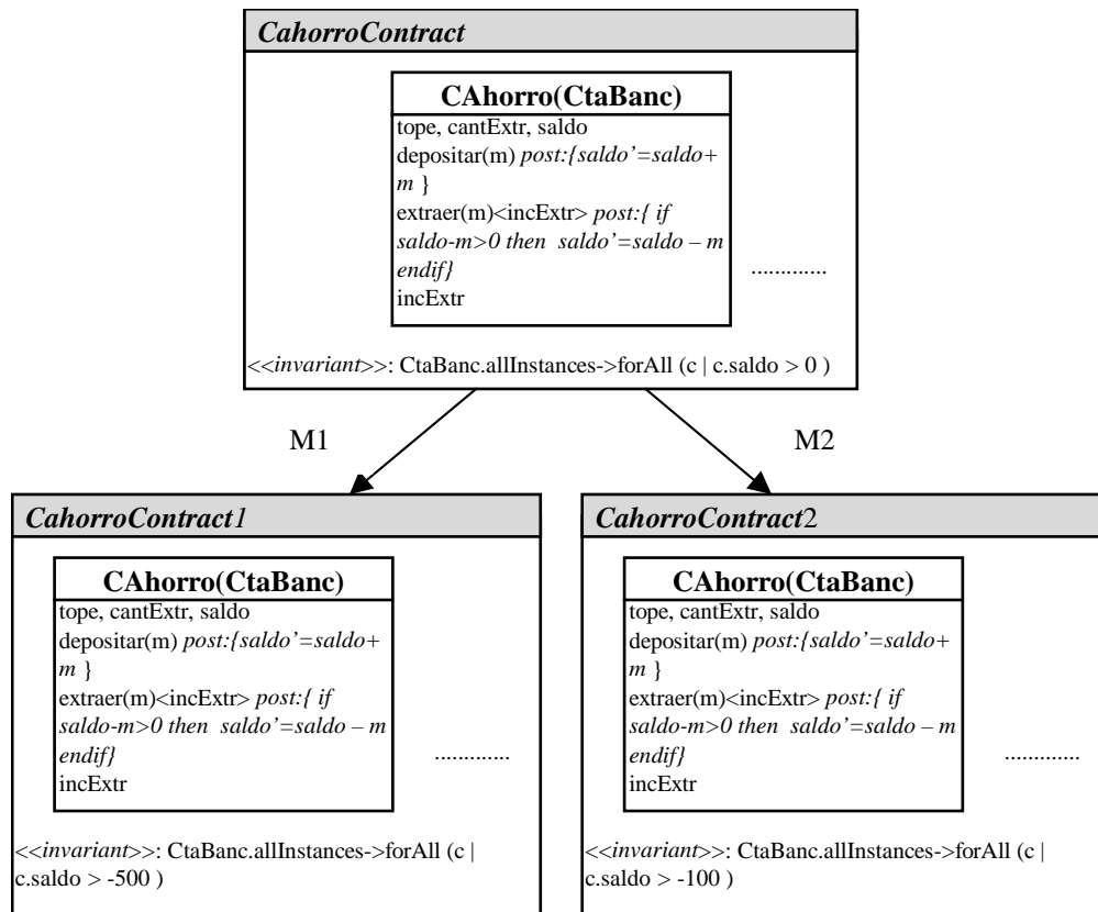
Fig 6.6 Incoherencia Semántica de Invariante
